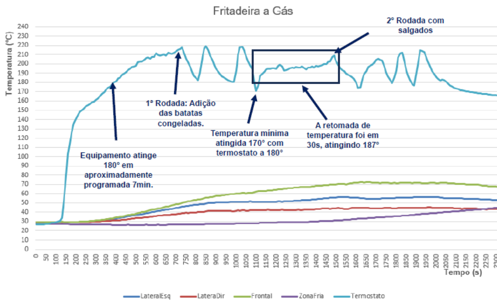
Gráfico 1: Aquecimento x Tempo – Fritadeira a gás.
